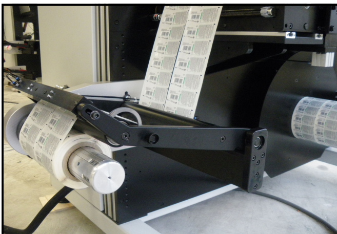
Pinza automática en rebobinado en rodillo pisador
